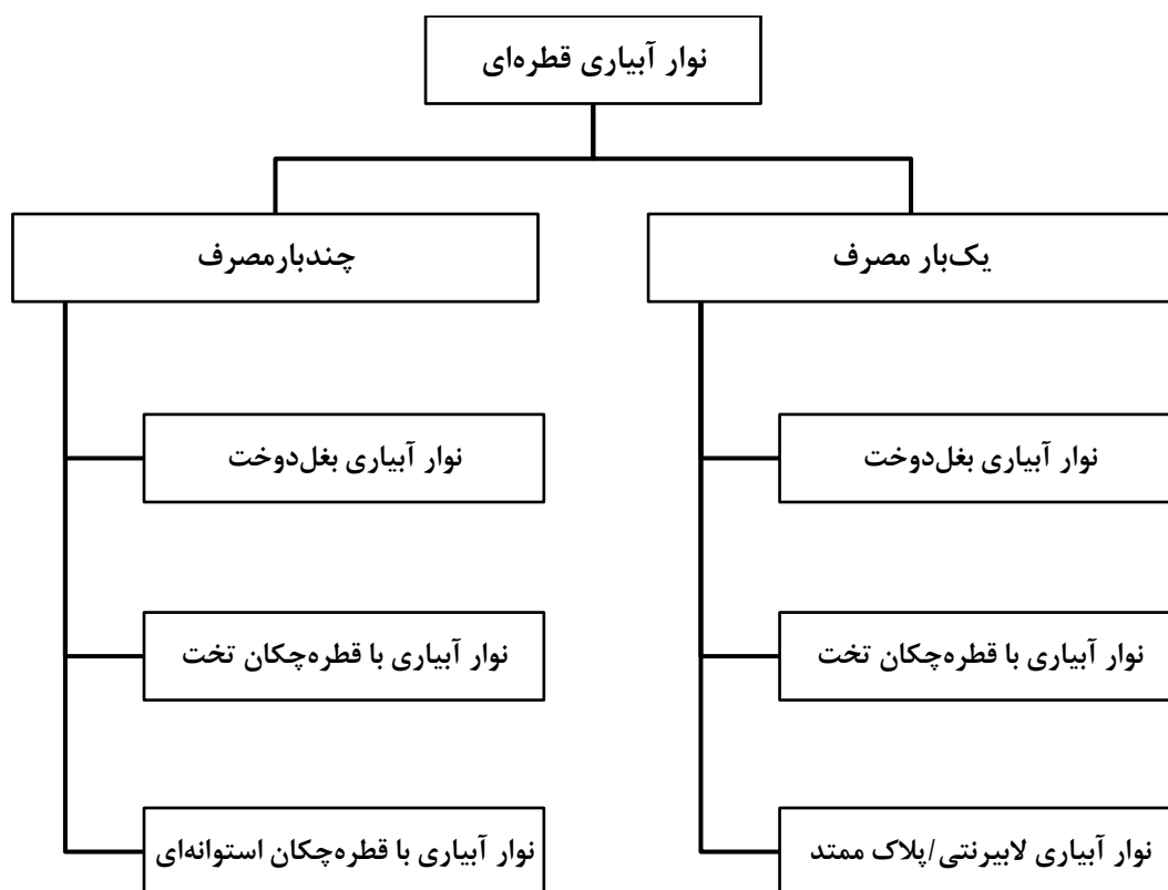
شکل ۱- انواع نوار آبیاری قطره‌ای یک‌بار مصرف و چندبار مصرف بر اساس فناوری تولید
